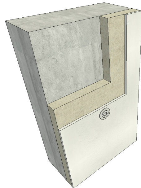
2 פרספקטיבה
