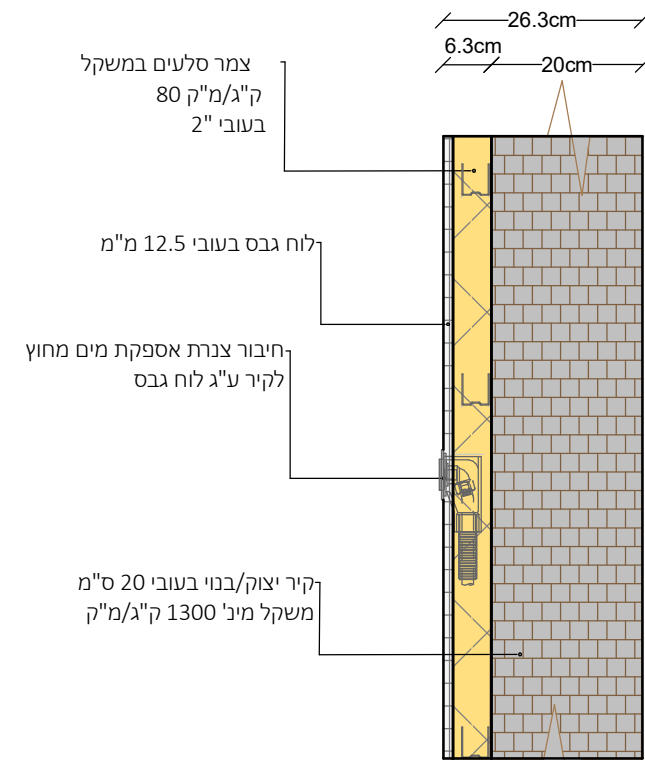
3 חתך 1:10
