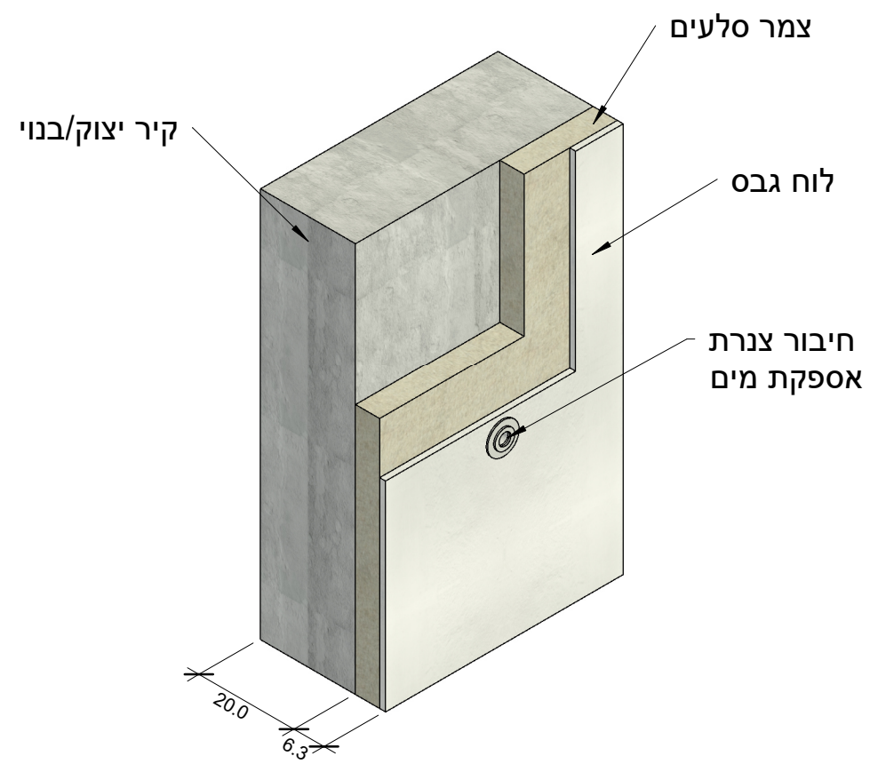
1 איזומטריה
